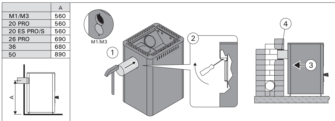
Рисунок 9. Присоединение каменки к каменному дымоходу через заднее соединительное отверстие (все размеры приведены в миллиметрах)
