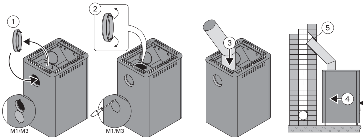
Рисунок 10. Присоединение каменки к каменному дымоходу через верхнее соединительное отверстие (все размеры приведены в миллиметрах)
