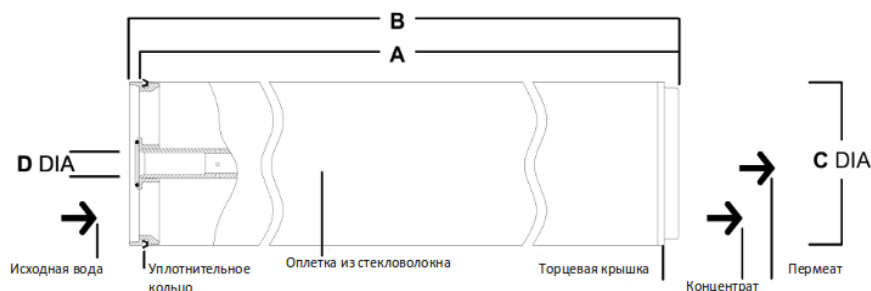
Габаритные размеры – дюймы (мм)
